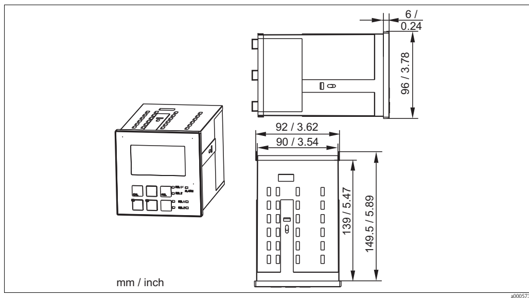
盘装型变换器的外形尺寸示意图
