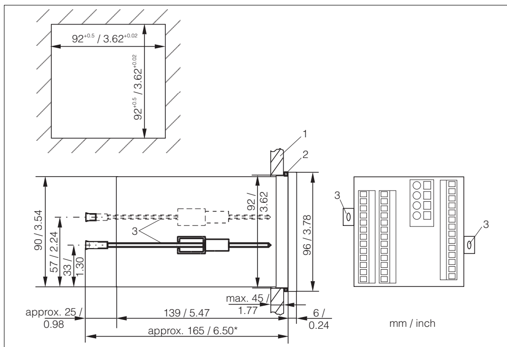
盘装型变换器的安装示意图
